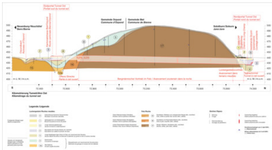
Geologisches Längsprofil Büttentunnel
